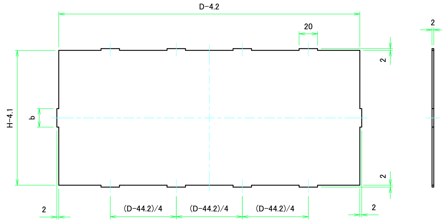
Dパネル1表面 / D panel 1 Frontside
